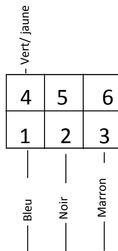
Connecteur moteur Male
